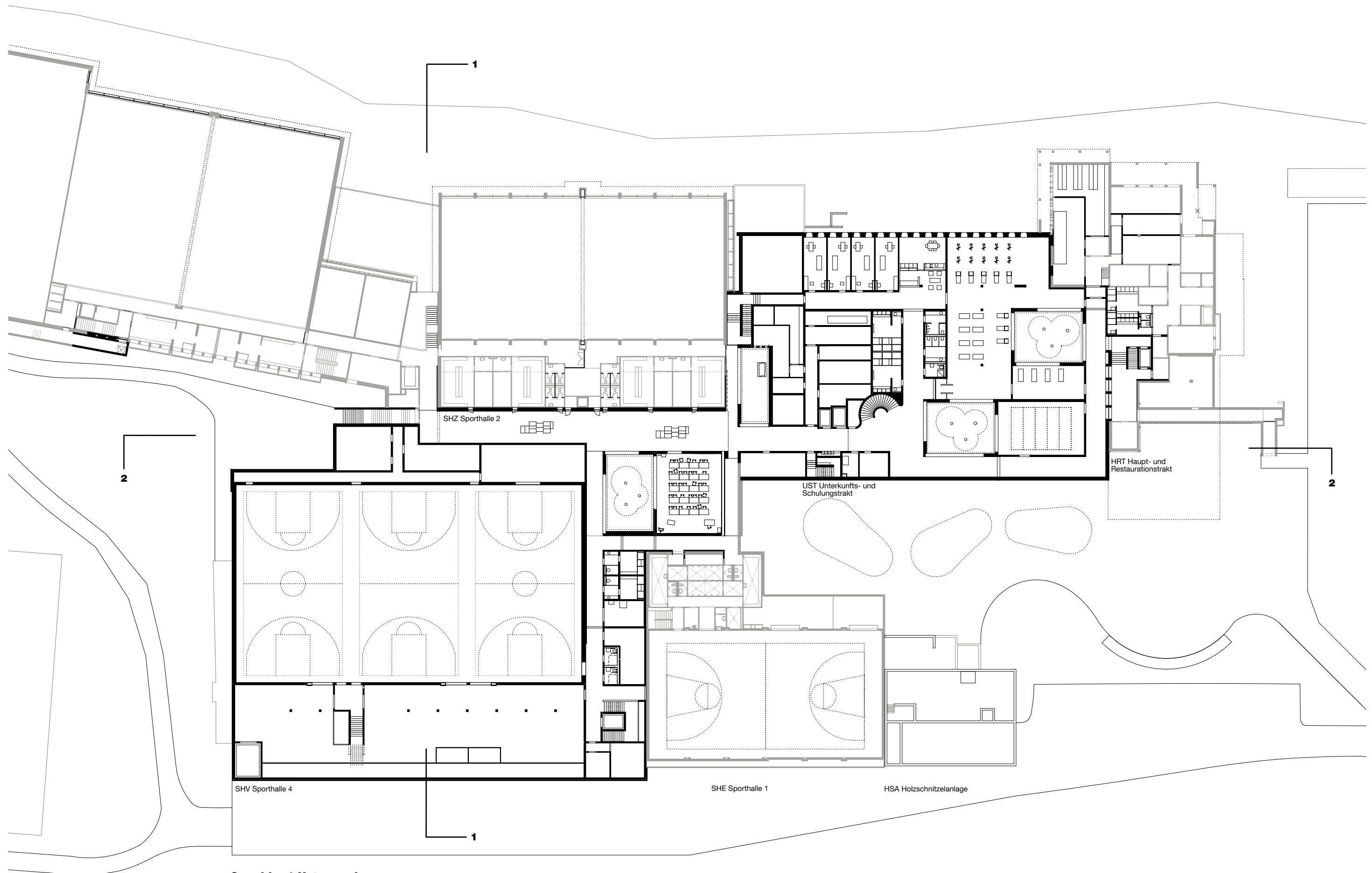
Grundriss 1. Untergeschoss
