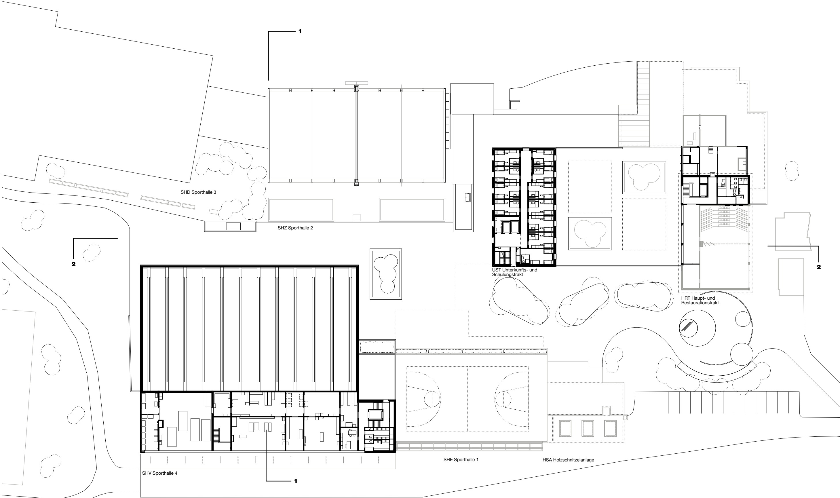
Grundriss 1. Obergeschoss
