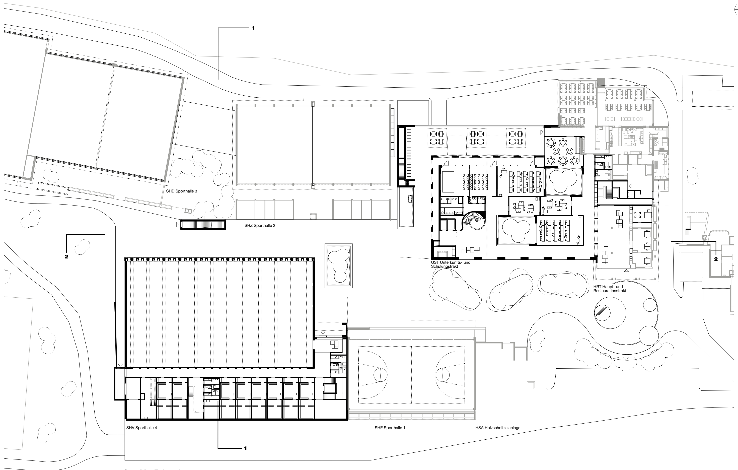
Grundriss Erdgeschoss
