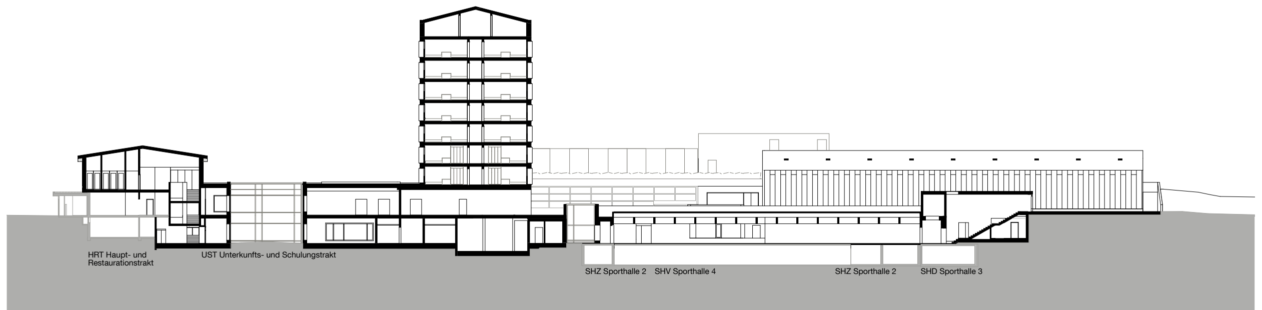
Schnitt 2-2
