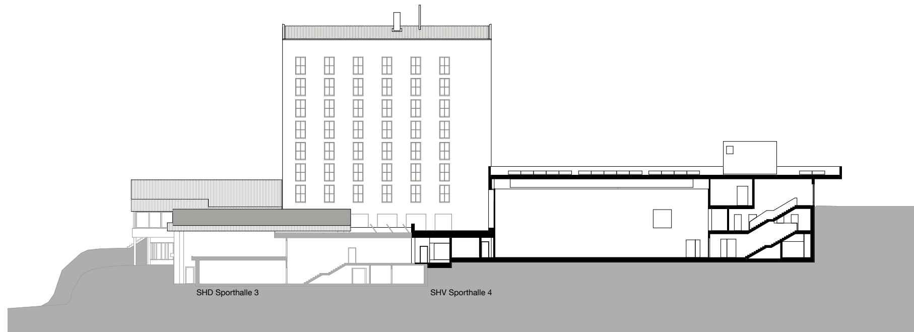
Schnitt 1-1
