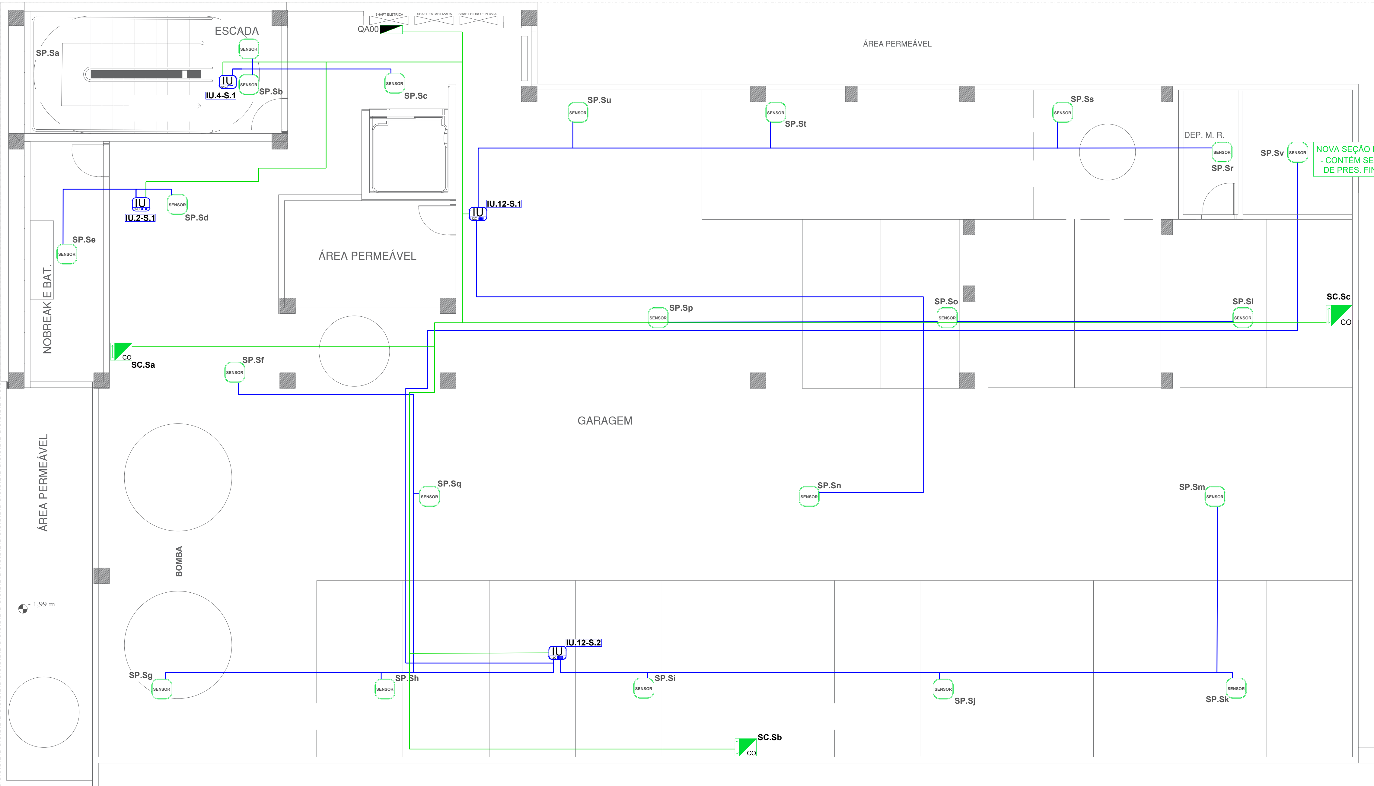
PLANTA BAIXA SUBSOLO
