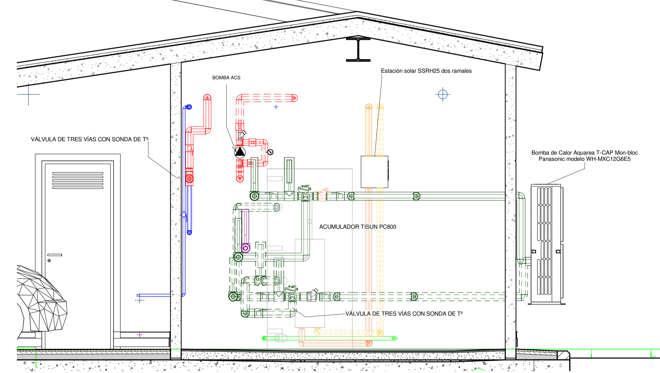
5 SECCIÓN 1 SALA MAQUINAS DETALLE ALTO Escala 1:25
