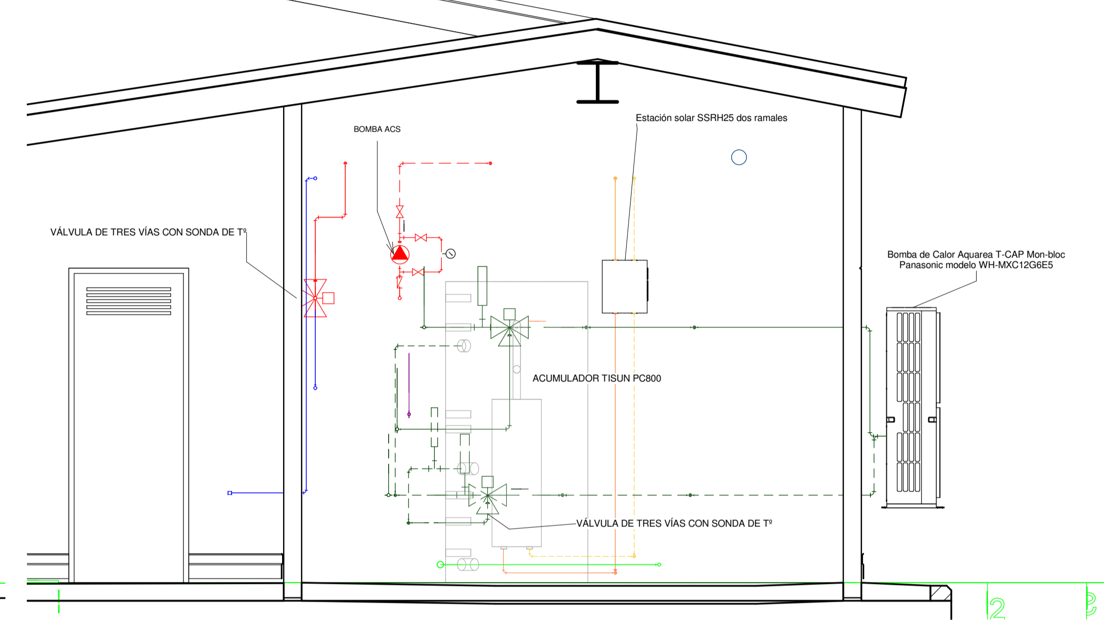
2 SECCIÓN 1 SALA MAQUINAS Escala 1:25
