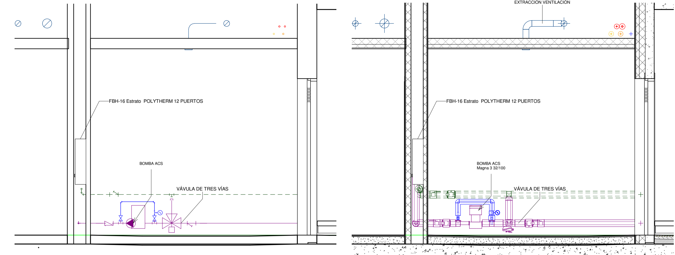
3 SECCIÓN 2 IMPULSIÓN Y RETORNO SUELO RADIANTE Escala 1:25
